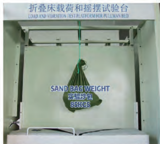
动载荷试验 | Dynamic Load Test
