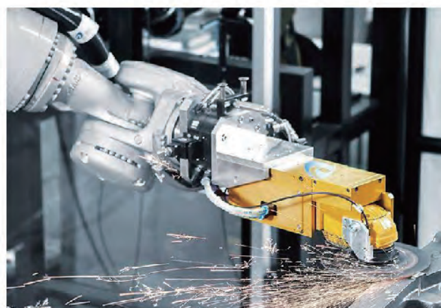
机械臂打磨 Mechanical-Arm Grind
